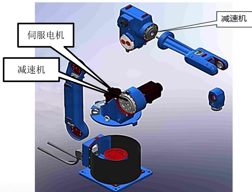
工業ロボット
