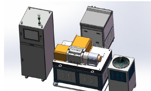
耐久试验机 Endurance Testing Machine
